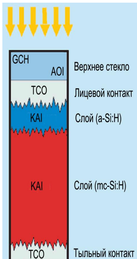
Структура солнечного модуля
